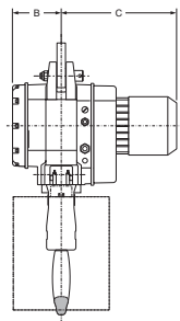
LK függesztőlappal
