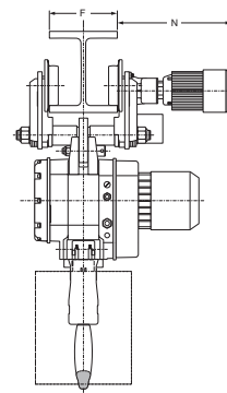
LK haladóművel
